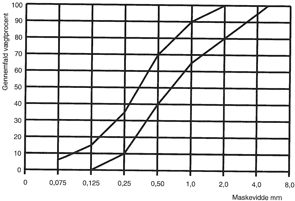
Grænsekurver for mørtelsand
